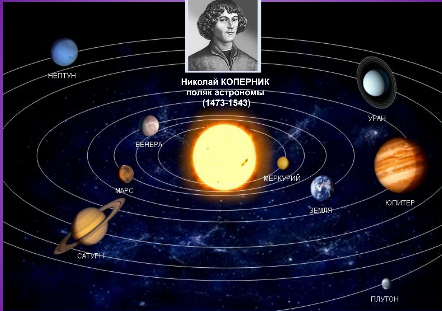
Күн жүйесі
