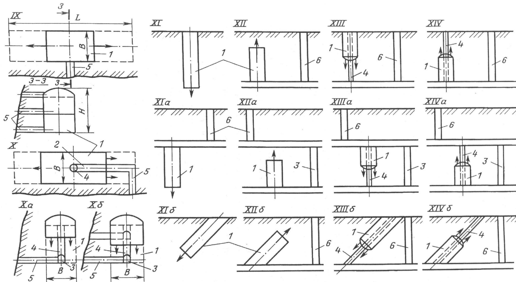
Рис. 3.6. Схемы строительства подземных сооружений:
