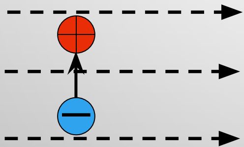
Полярная молекула
