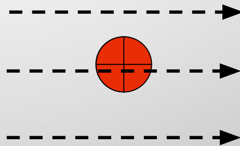
Неполярная молекула
