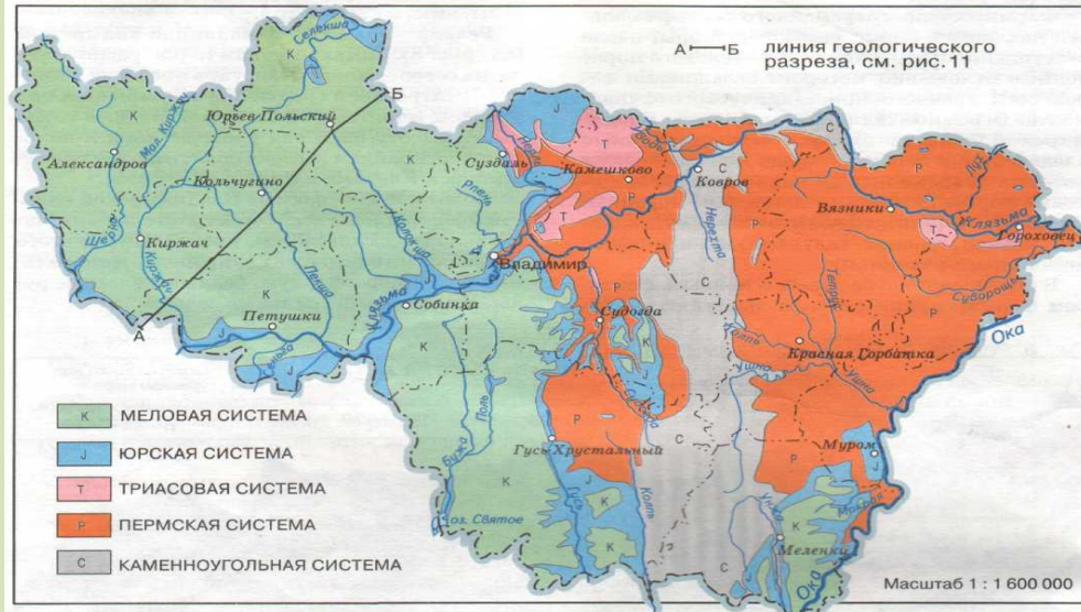
Рис. 10. Геологическое строение
