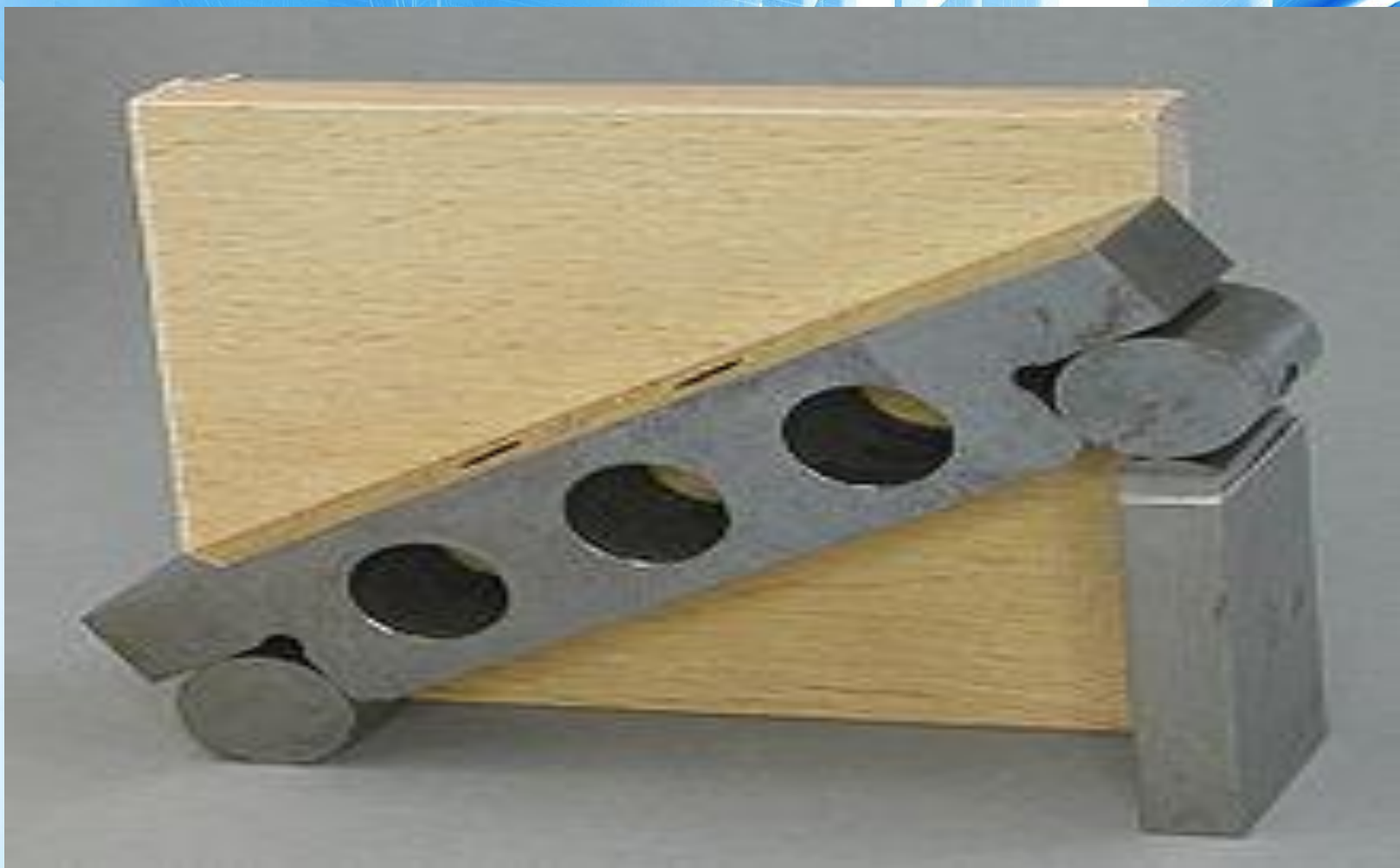
Синусная линейка
