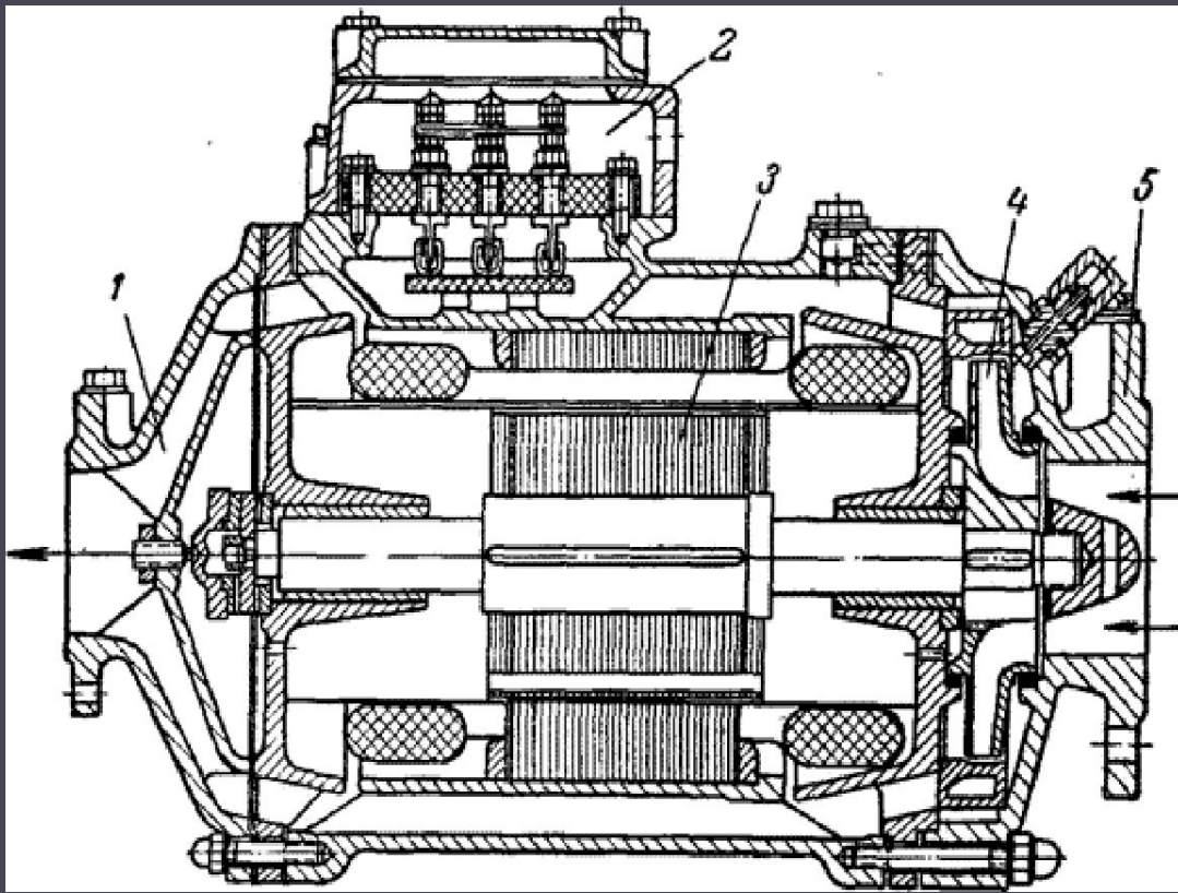
Центробежный угловой насос
