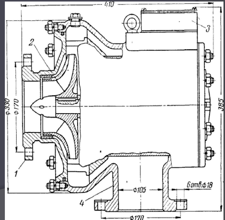
Центробежный угловой насос
